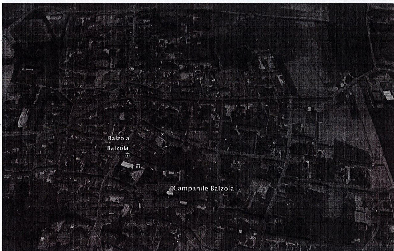
Figura 2: Mappa di copertura radioelettrica dalla Postazione 2 (Balzola, Campanile)
