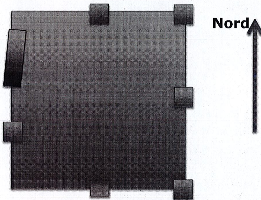
Figura 9: Collocazione degli impianti trasmettenti all'interno della cella campanaria. In rosso le antenne di distribuzione del segnale (con radio integrata). In nero il collegamento verso la postazione 1.
